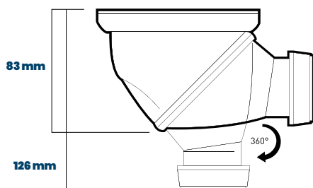
bonde 360° orientable
