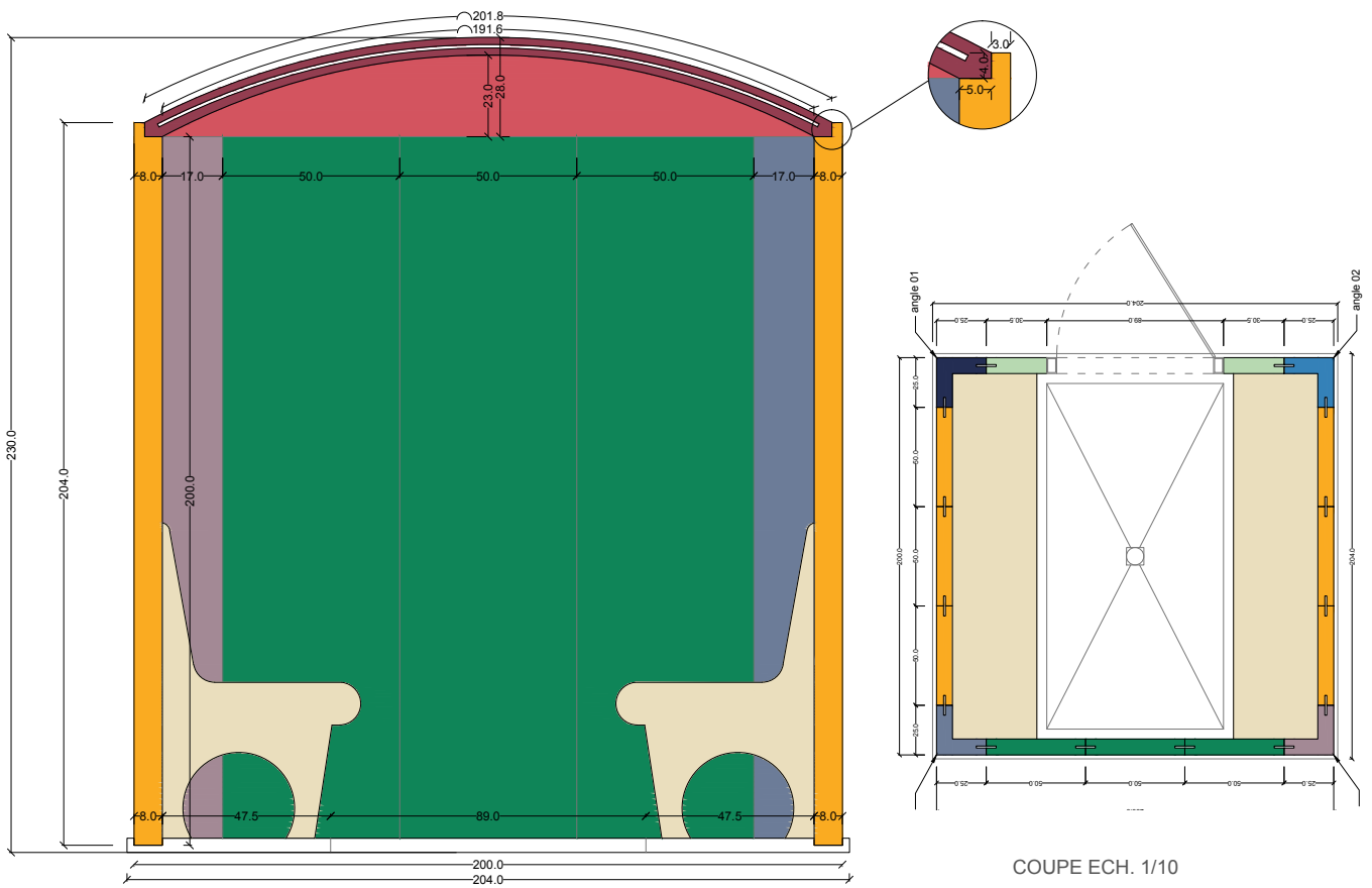
Exemple de plan Plans réalisés sur mesure par un architecte
